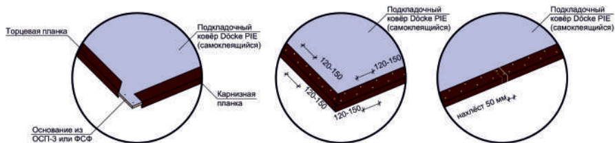
Рис. 8 Крепление металлических карнизных и торцевых планок.
