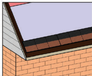
Рис. 11 Схема укладки коньково-карнизной черепицы на карнизе.
